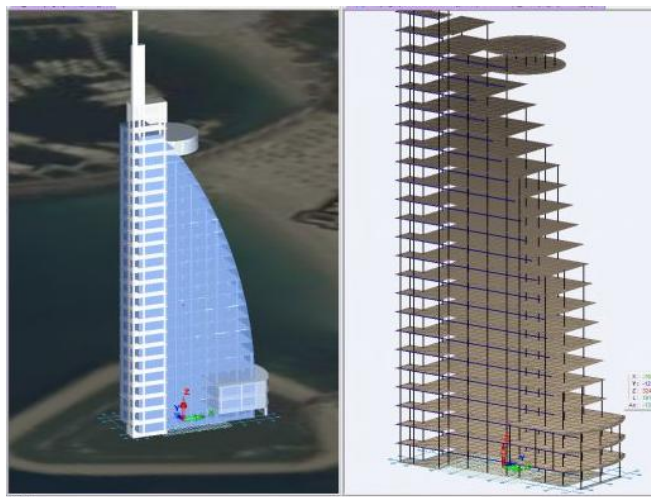
Рис. 4. Пример создания модели здания по концептуальным формам
