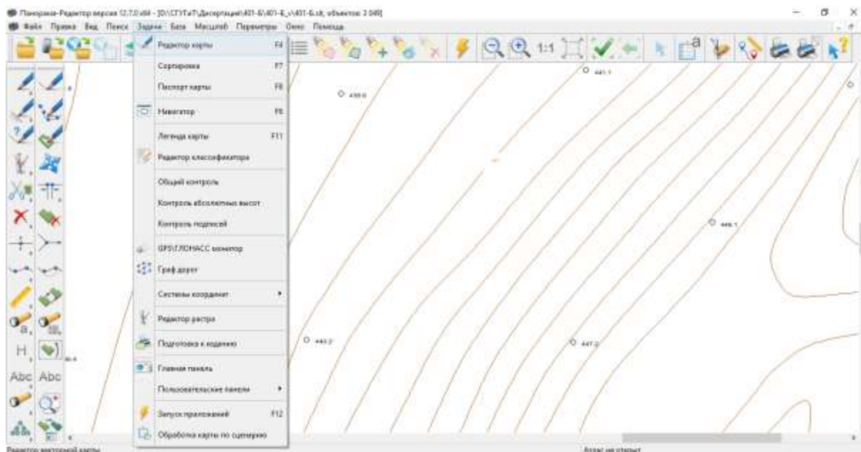
Рис. 3. Редактор карты
