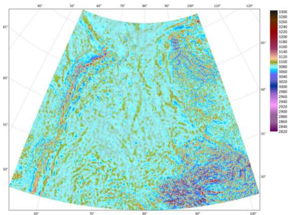
Рис. 1. Картограмма вычисленных ВГСТ на территории Западной Сибири (в Этвешах)
