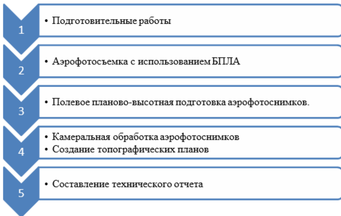
Рисунок 3 – Технологическая схема выполнения работ при создании цифровых топографических планов
