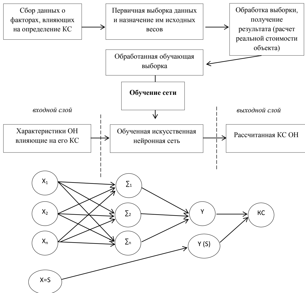
Рисунок 1 – Схема работы искусственной нейронной сети
